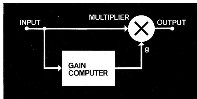
Vorwärts-Regelung
